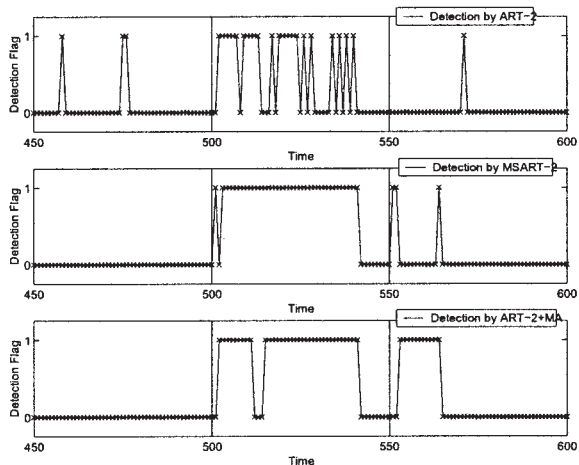
(d) ART-2 and MSART-2 Detection Performances
